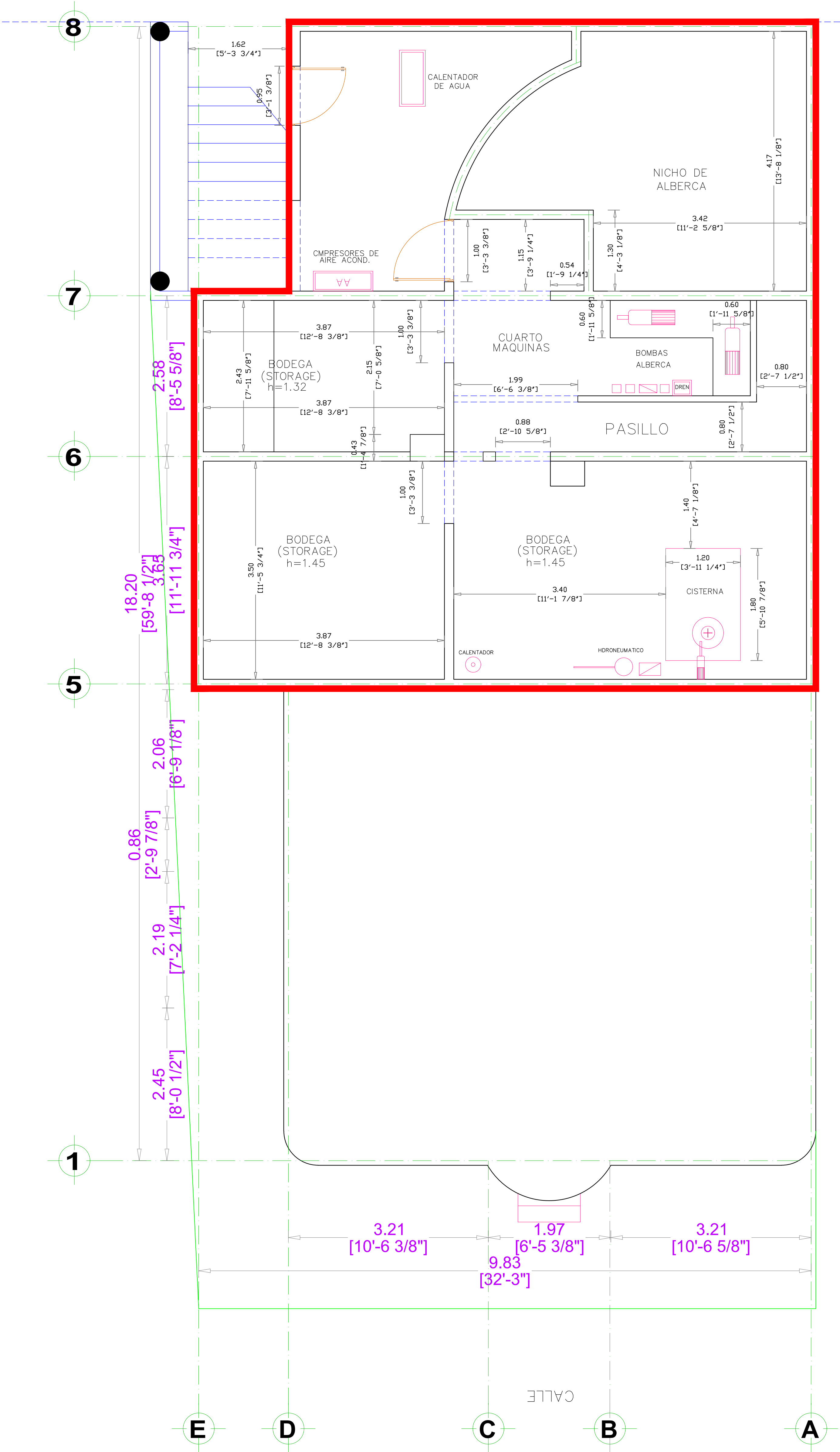
Planta Arquitectonica Sotano
